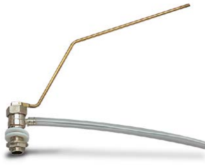
FLOTADOR SILENCIOSO VERTICAL Con asiento anticorrosivo. En latón fundido, con varilla angular. NOISELESS VERTICAL FLOAT With anti-corrosion seating. In cast brass, with angle rod.
